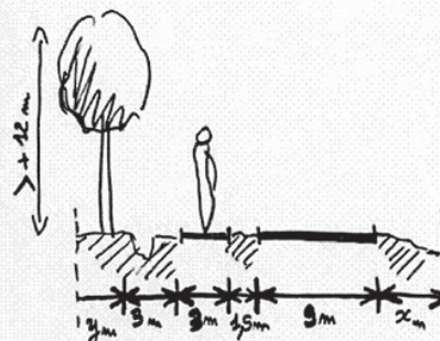
Exemple de coupe sur voirie en plan masse du règlement
